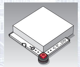
90°-Aussenwinkel
