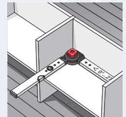
90°-Innenwinkel
